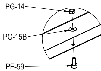
DÉTAIL B ECHELLE 1 : 3
