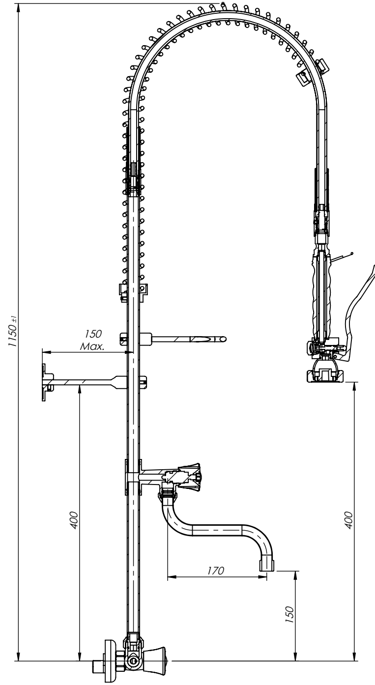
A-A Kesiti
