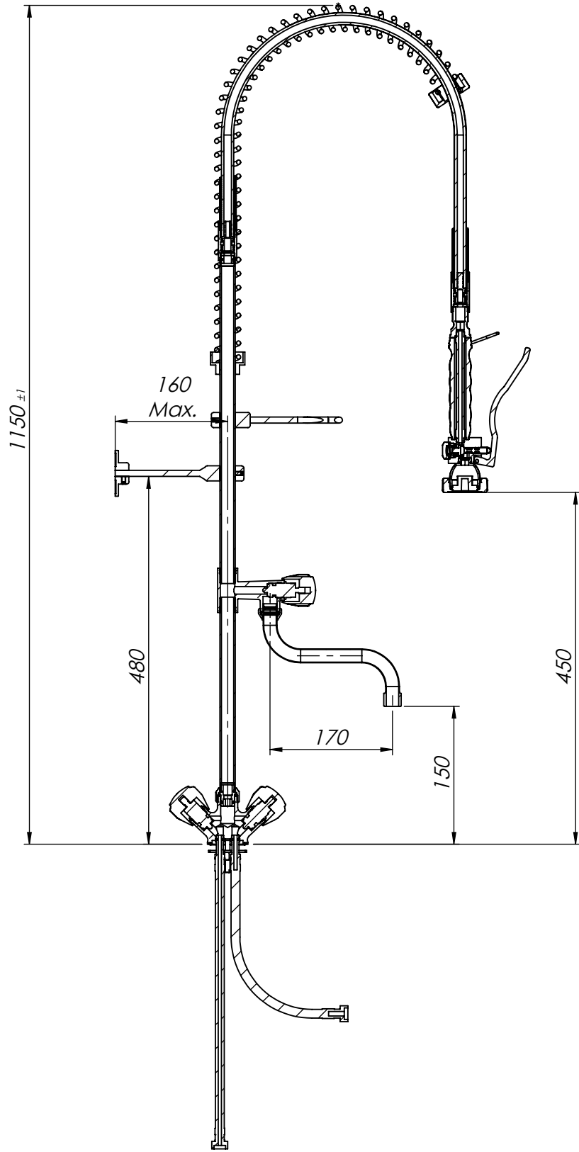
A-A Kesiti (1 : 7)
